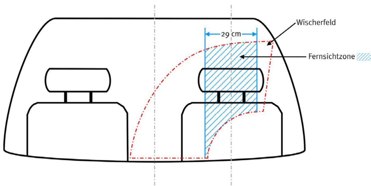
Fernsichtfeld des Fahrers
